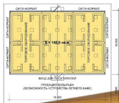
ПЛАН НЕСТАЦИОНАРНОГО ТОРГОВОГО ОБЪЕКТА
